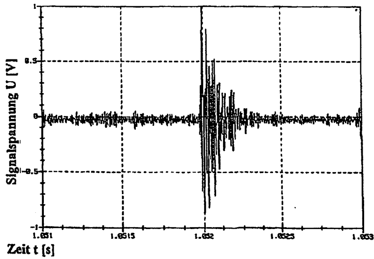
Burstsignal der Schallemission bei Rißbeginn im menschlichen Knochen
